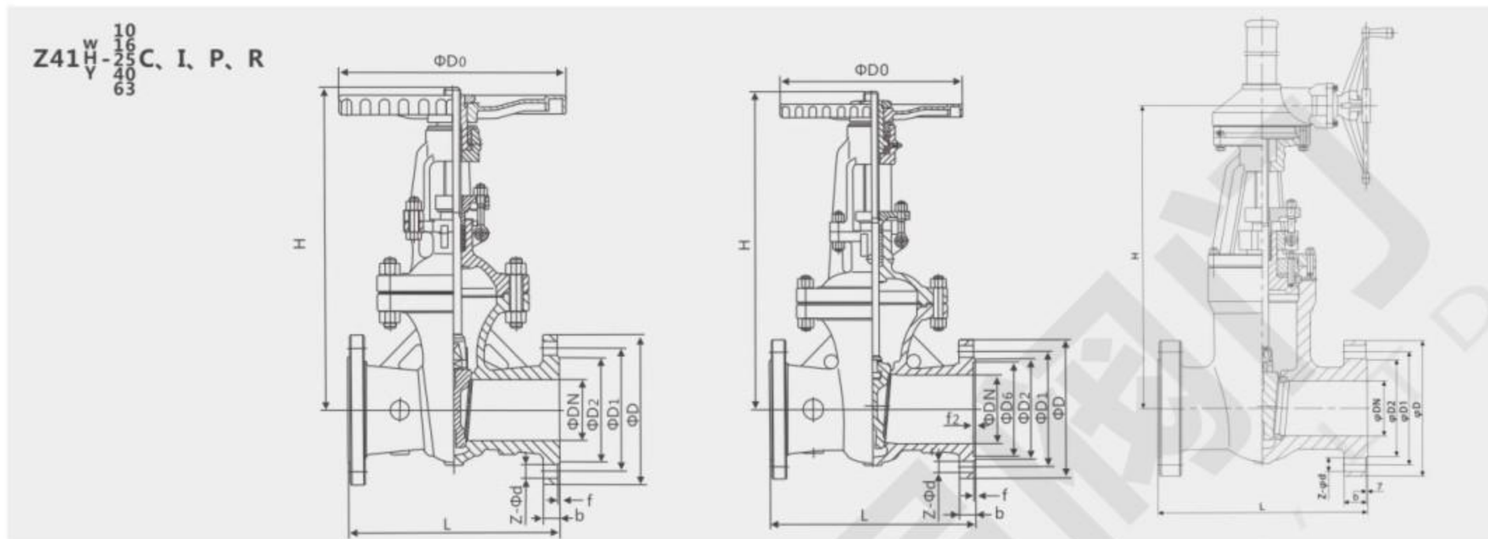
PN10 国标法兰闸阀
